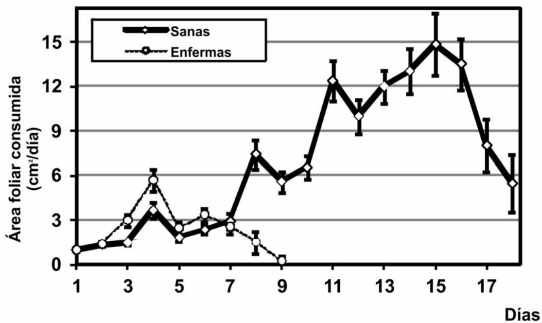
Figura 3. Evolución de la tasa diaria de consumo foliar de larvas de S. frugiperda sanas e infectadas con VPNSf aislamiento Leales, a los tres (a) y siete (b) días de nacidas. Se indican los valores promedio de la muestra de larvas sanas e infectadas evaluadas; las barras indican el error estándar.
